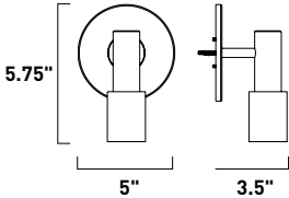
E21720-BK, -GM Spot Light
