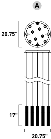
E11019-144BK, -144GLD Pendant
