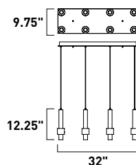
E24758-BKGLD, -SNSBR Pendant
