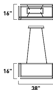
E21266-BK, -GLD Pendant
