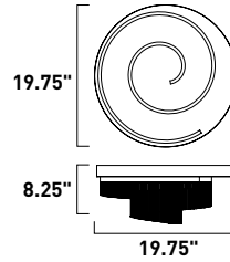
E24778-133BK Flush Mount
