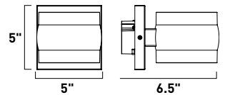
E30171-10BK Interior/Exterior Wall
