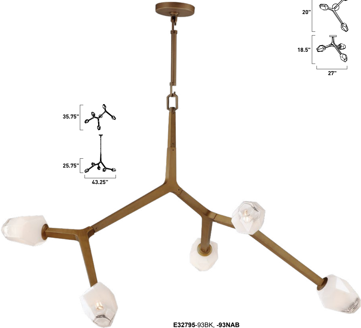
E32795-93BK, -93NAB Pendant
