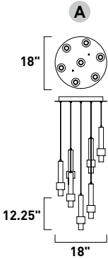
E24757-BKGLD, -SNSBR Pendant
