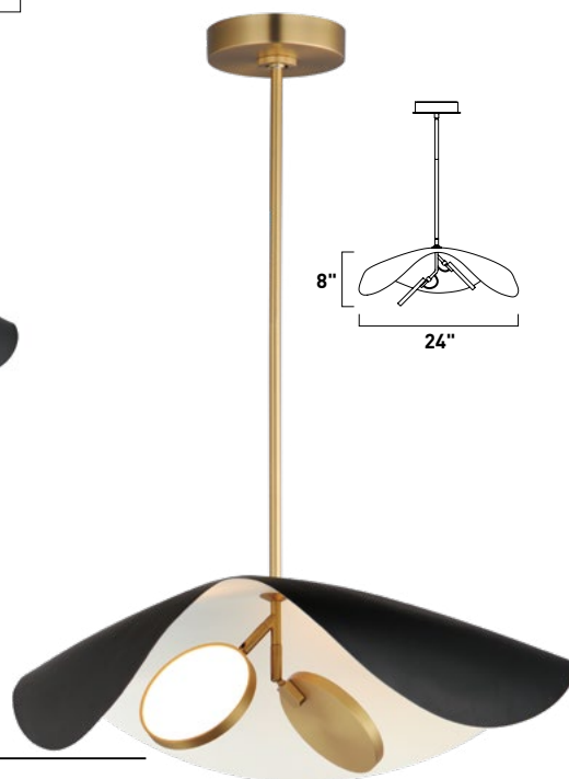
E24966-WTBK, -WTBKGLD Pendant
